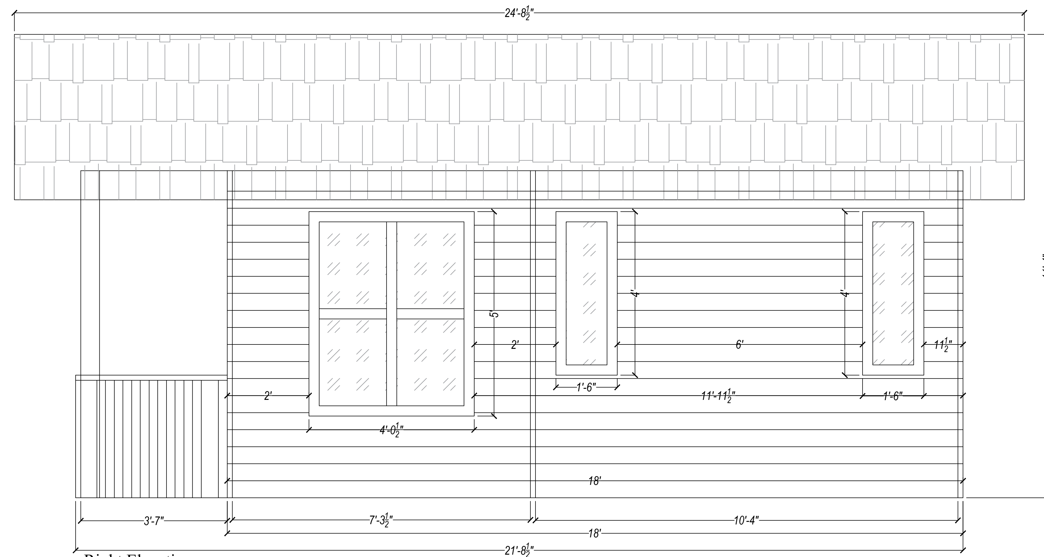
Right Elevation
